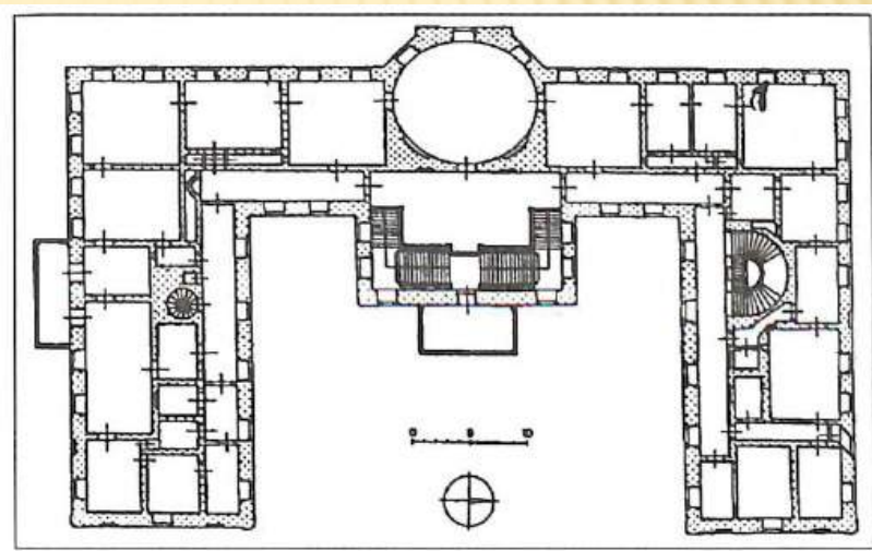
Půdorys napajedelského zámku (konec 19. století)
